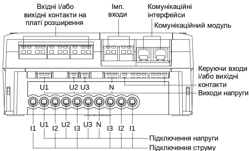
Рисунок 8 – Зовнішній вигляд колодки затискачів лічильника ZMDxxx
