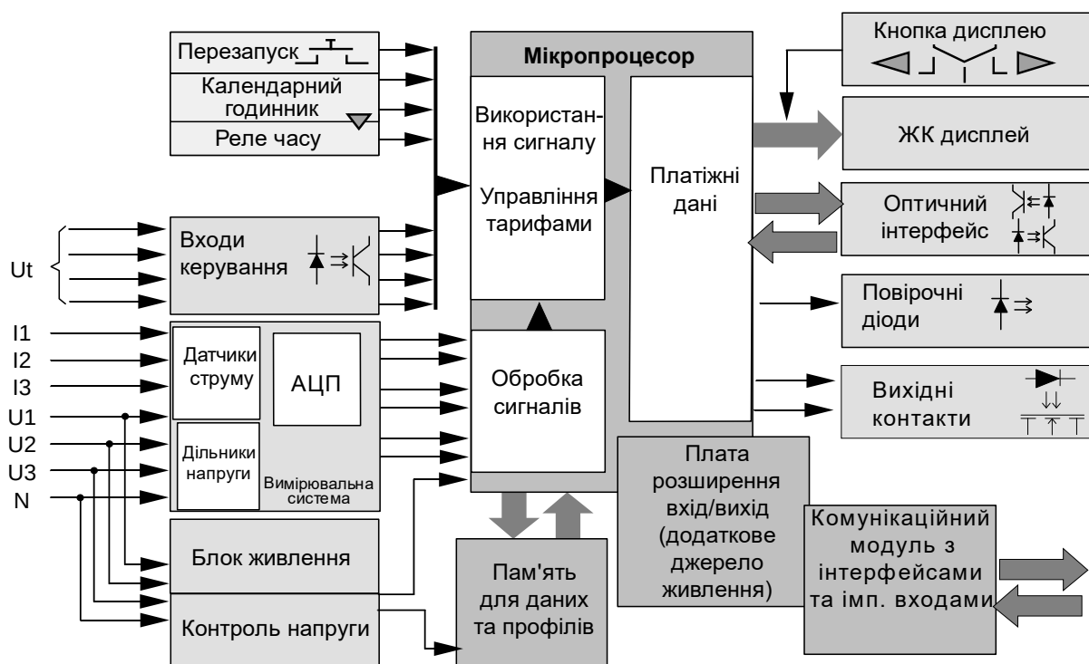
Структурна схема
