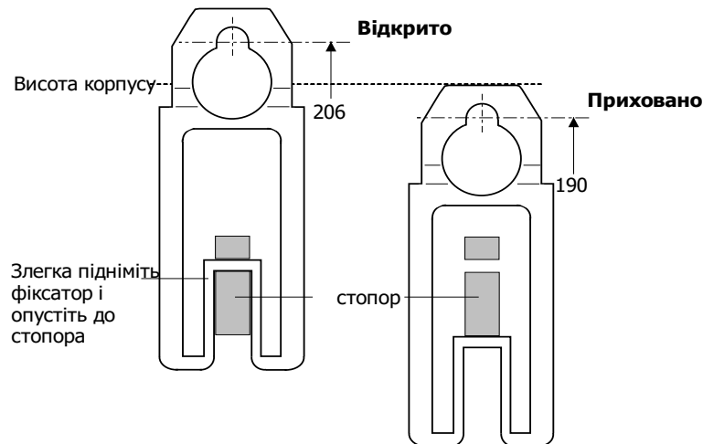
Рисунок 9 - вушко для кріплення (відкрите або приховане)
