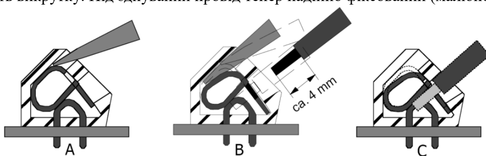
Рисунок 12 - Підключення в гвинтові підпружинені клеми
