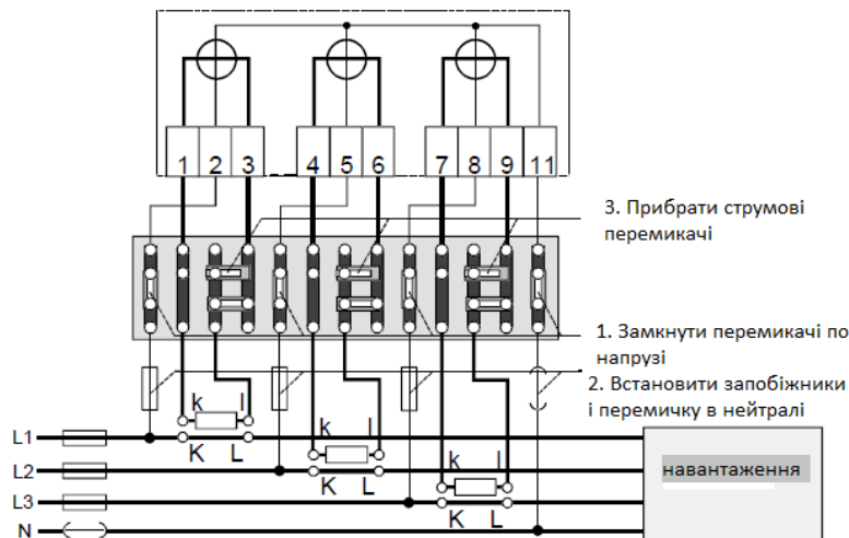
Рисунок 13 – Положення клемного терміналу після вводу в експлуатацію
