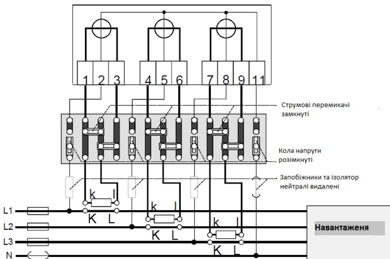
Рисунок 11 – Стан клемного термінала перед встановленням лічильника
